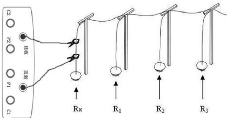
图 3 多点接地系统地阻的测量
