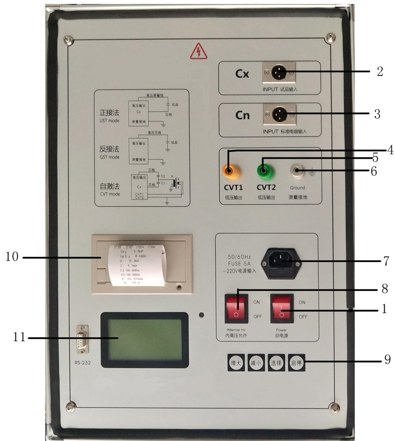
面板示意图(图片仅供参考, 以实物为准)
