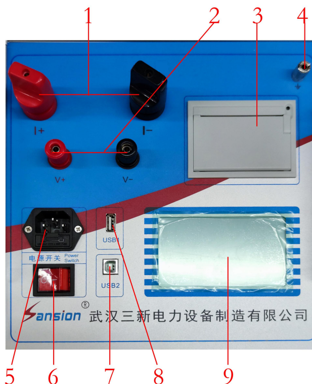
图一 回路电阻测试仪面板（图片仅供参考，具体以实物为准）
