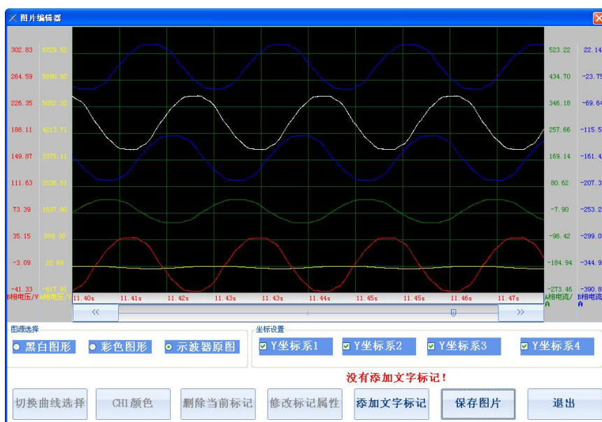
图 24 图形编辑
