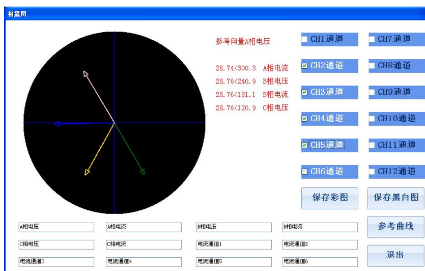
图 29 相量图工具
