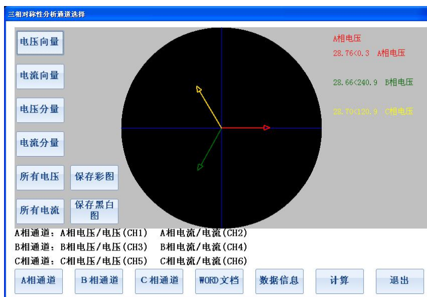
图 28 三相分析相量图
